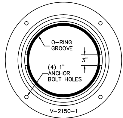
MANHOLE FRAME
