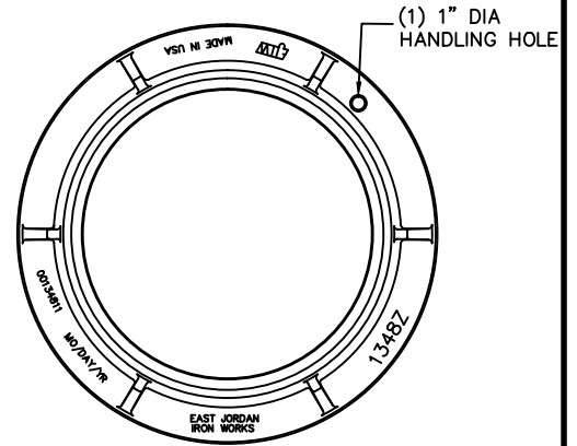
MANHOLE FRAME
